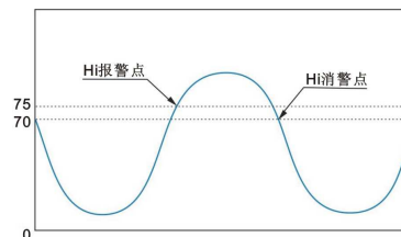
图 5-8 上限报警回差
