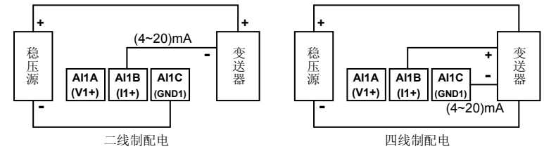
(e)变送器配电接线图（外接 24V 稳压源）
