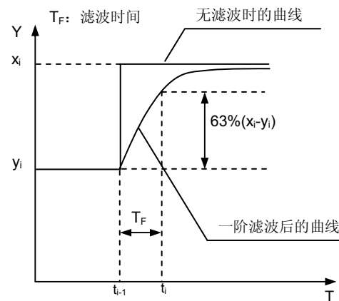
图 5-5 一阶滤波
