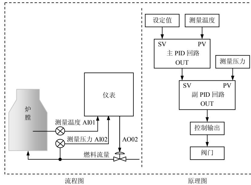
图 6-6 串级控制
