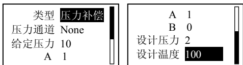
图 7-6 线性压力补偿组态画面
