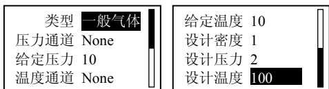
图 7-5 一般气体补偿组态画面
