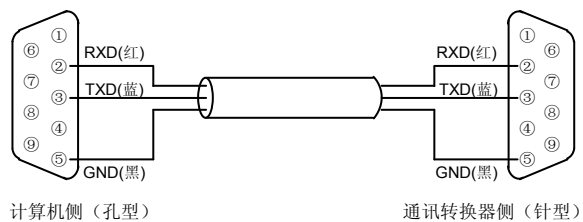
图 2-10 通讯转换器和计算机之间连接示意图
