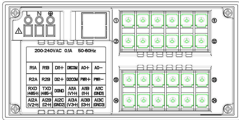
图 2-5 端子视图
