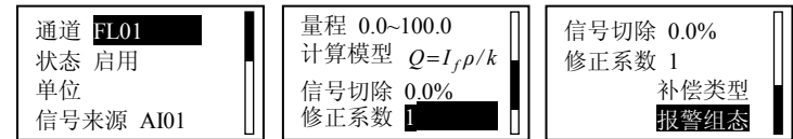
图 7-1 流量运算组态画面
