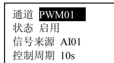
图 5-12 时间比例输出组态画面
