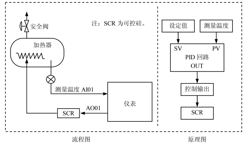
图 6-5 单回路控制
