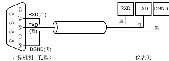
图 2-8 仪表和计算机 RS-232C 通讯连接示意图
