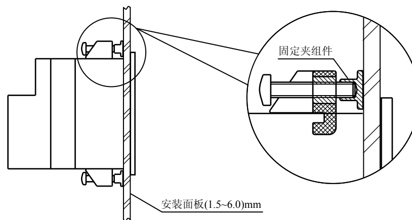
图 2-3 仪表安装
