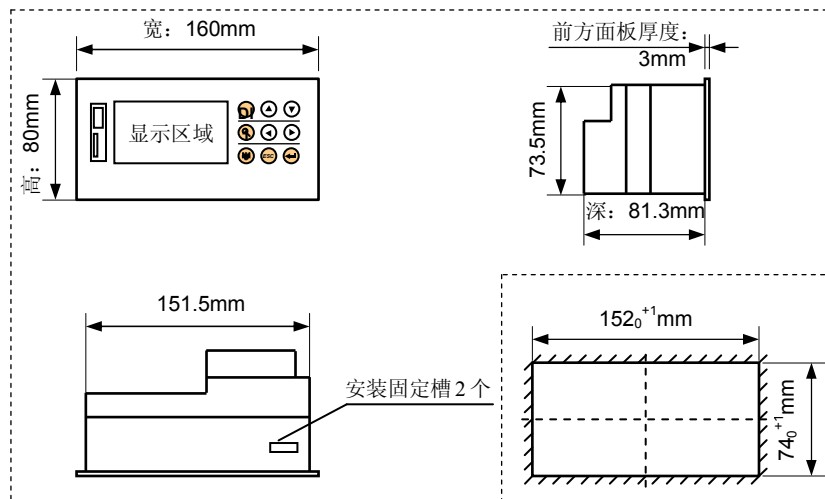
图 2-2 安装尺寸
