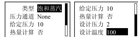
图 7-4 饱和蒸汽补偿组态画面
