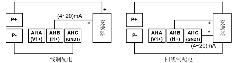
(d)变送器配电接线图
