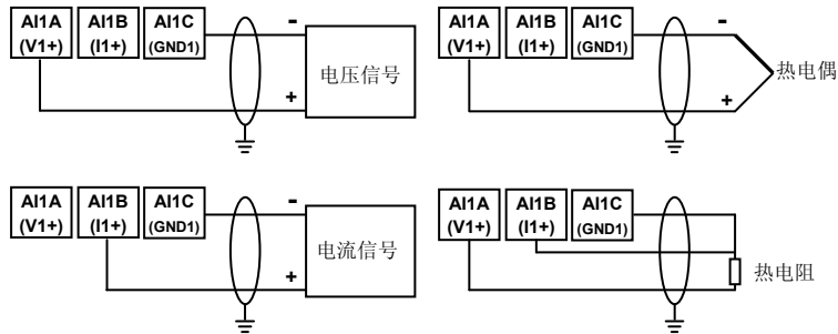
(a)模拟量输入信号接线图
