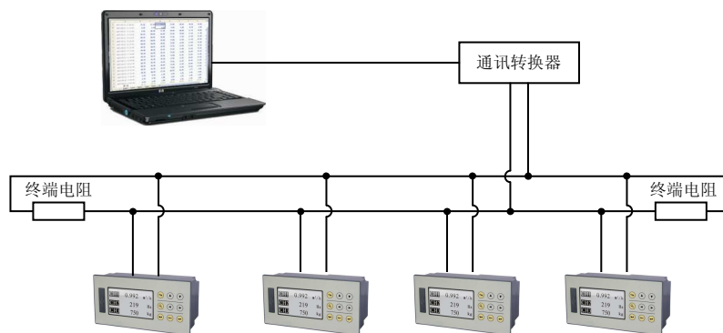
图 2-9 RS-485 通讯线的连接示意图
