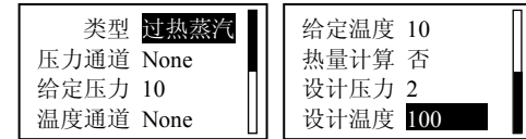
图 7-3 过热蒸汽补偿组态画面
