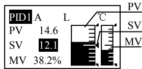
图 6-4 PID 控制画面
